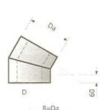
Bogen 30°
