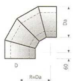
Bogen 90°
