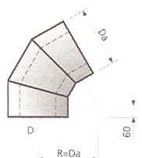
Bogen 60°
