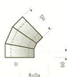
Bogen 45°
