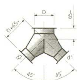
Hosenrohr 45°
