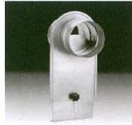
Beidseitig mit Stützen + Sicken, Arretierung mit Sterngriff
