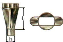
Übergänge oval-rund symmetrisch
