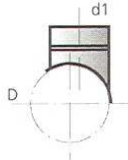
Sattelstück 90° exzentrisch
