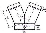
Hosenrohr 45° Culotte 45°
