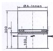
Deckenfutterrohr
